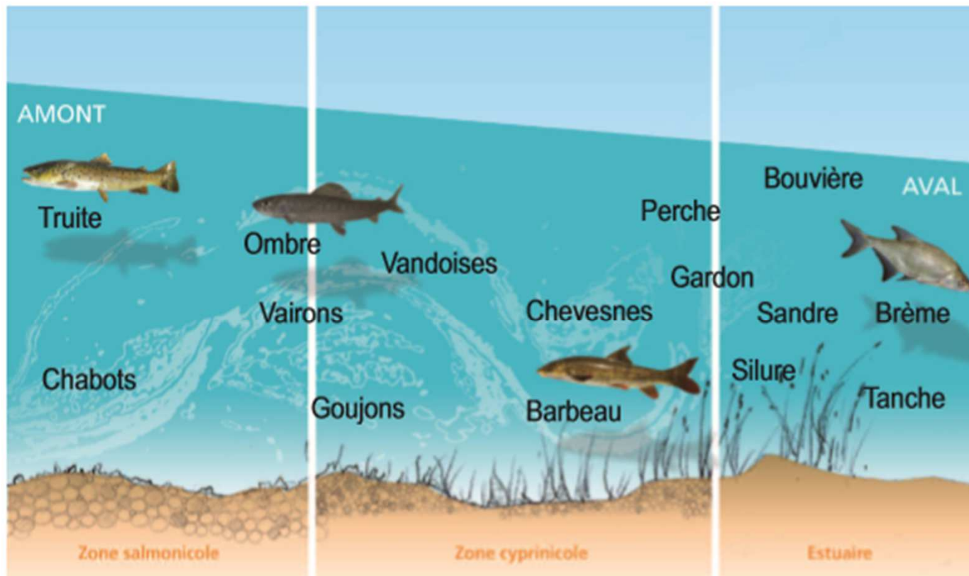
Évolution schématique de la structure des communautés piscicoles le long du gradient amont-aval.
